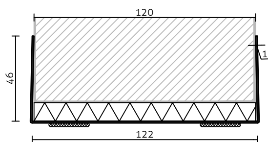
U profiel 120
