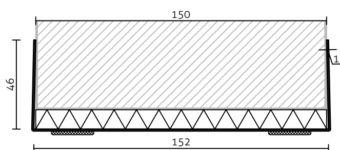
U profiel 150
