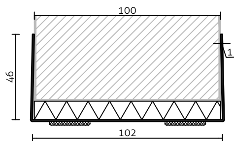
U profiel 100
