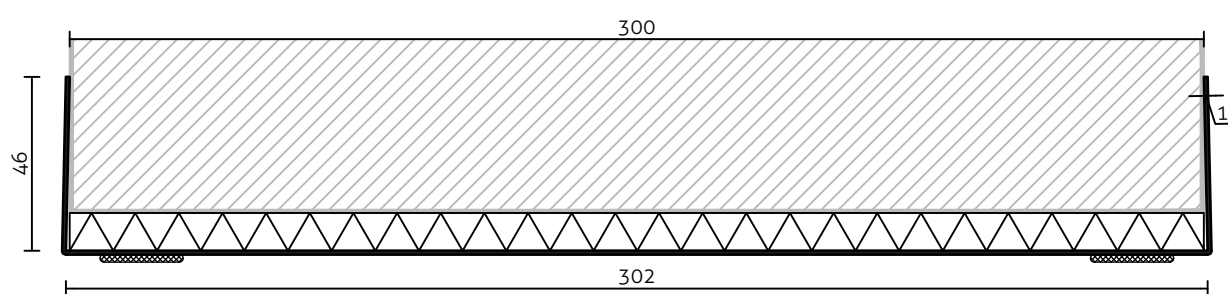
U profiel 300
