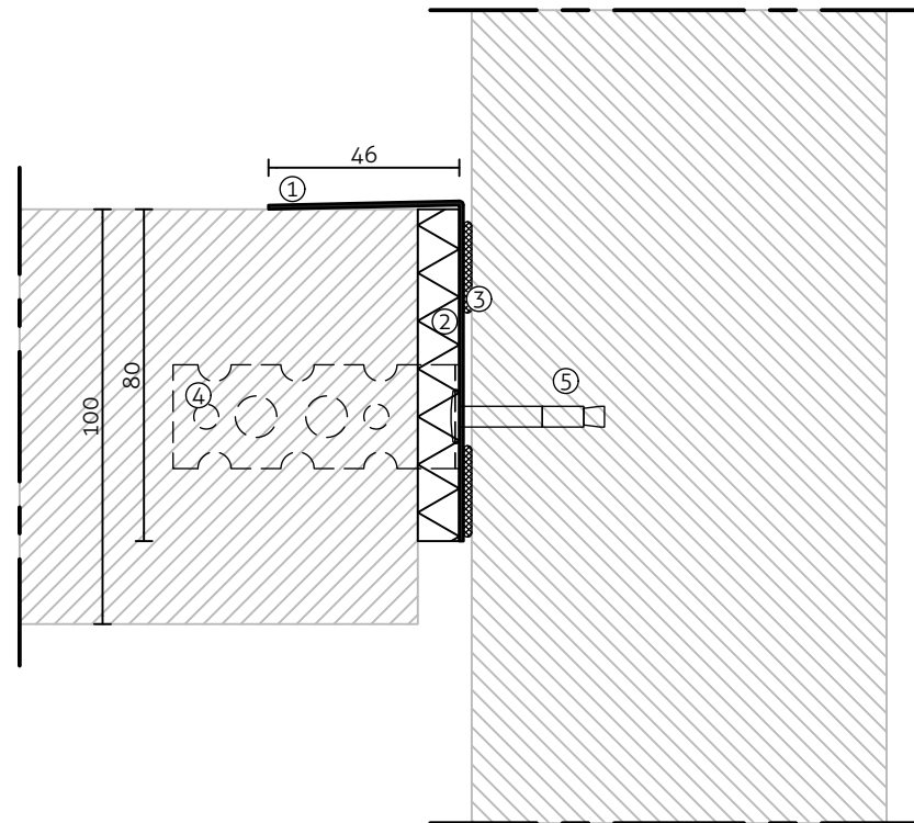
Safeprofiel wandaansluiting d.m.v. L-profiel
