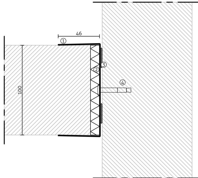
Safeprofiel wandaansluiting d.m.v. U-profiel
